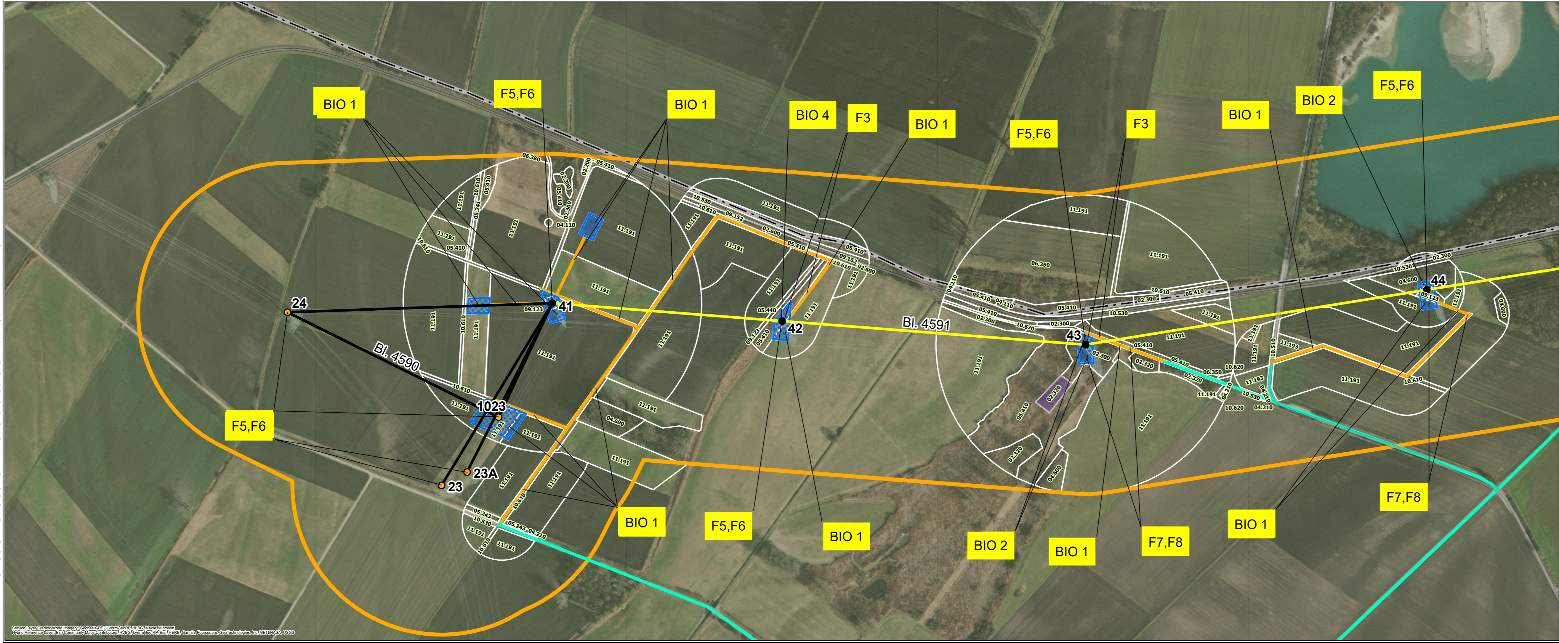
Legende siehe 5.2.5, 5.2.6 und 5.2.7 Tiere, Pflanzen und die biologische Vielfalt - Legende
